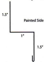
Double Angle (Z-Trim) Length 10'2"
